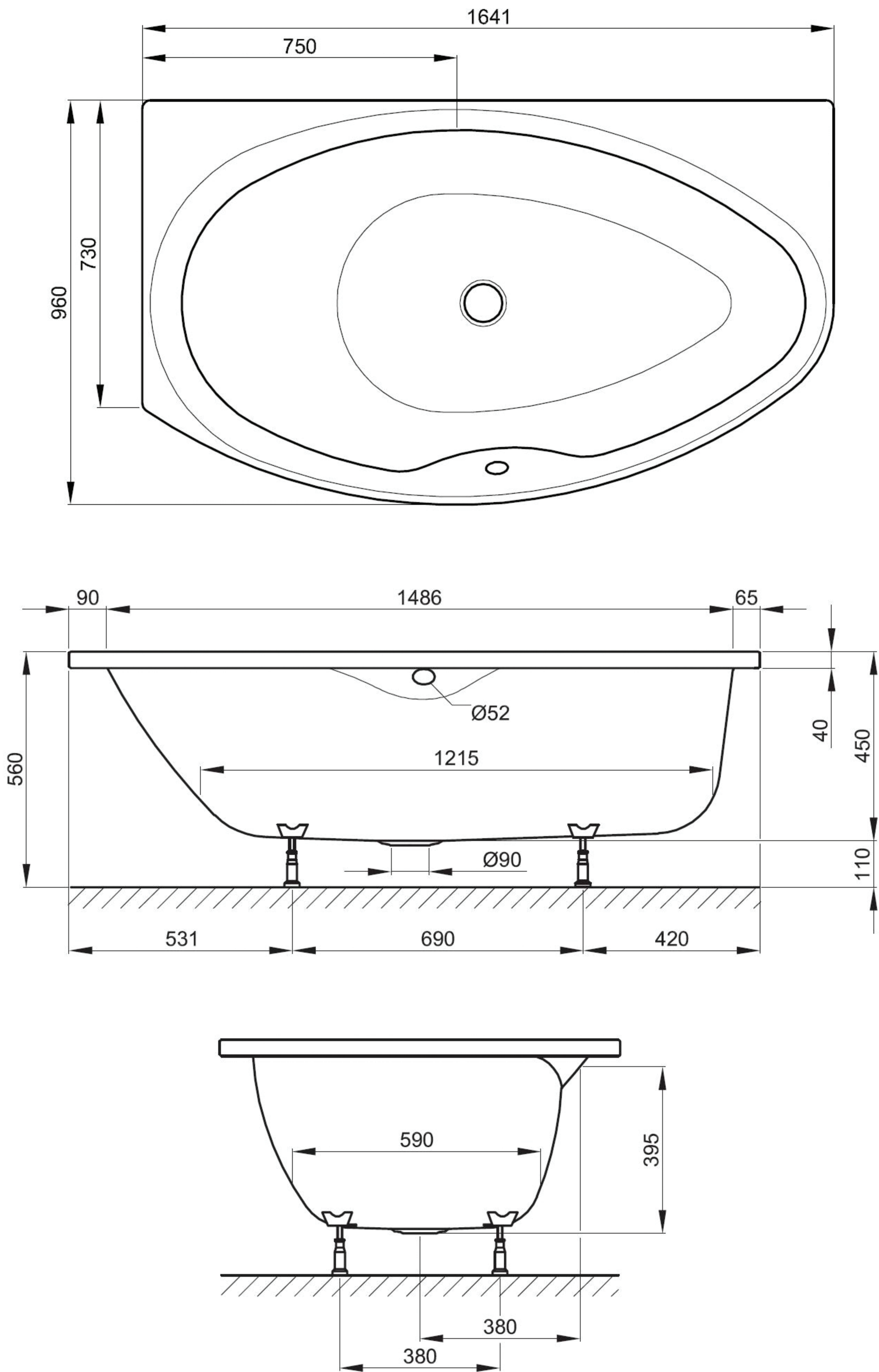
Výkres: Roh vlevo, obj. č. 6054
