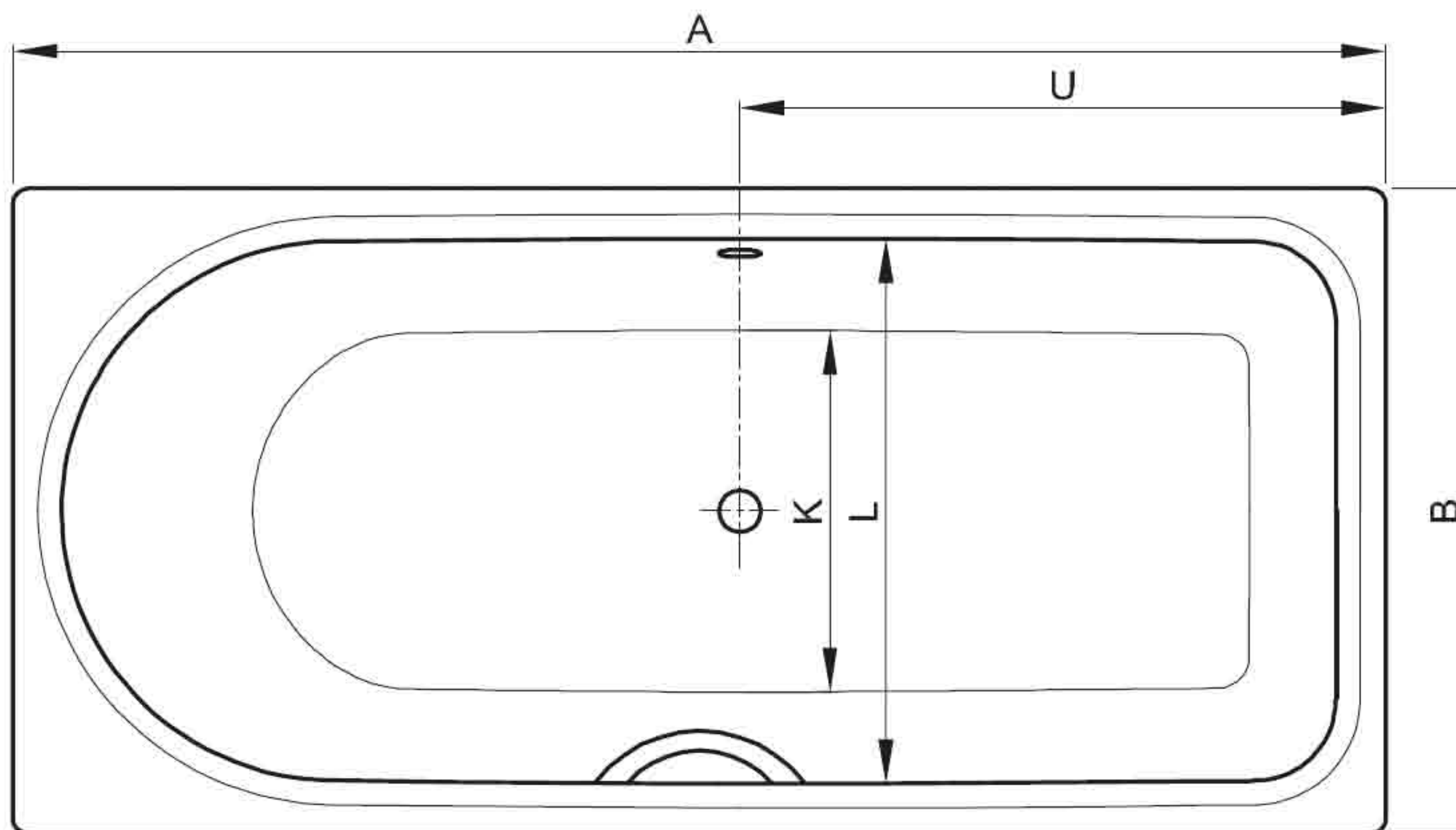
Výkres: Strana nohou vpravo, přepad vzadu, obj. č. 8830, 8832, 8834, 8836, 8838
