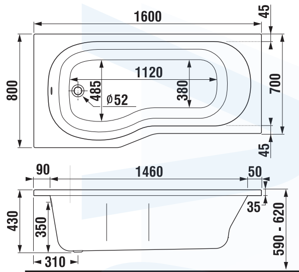
Instalační rozměry vestavné vany
