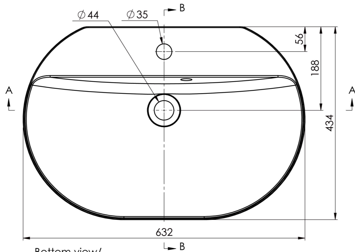
Bottom view/ Widok od dołu
