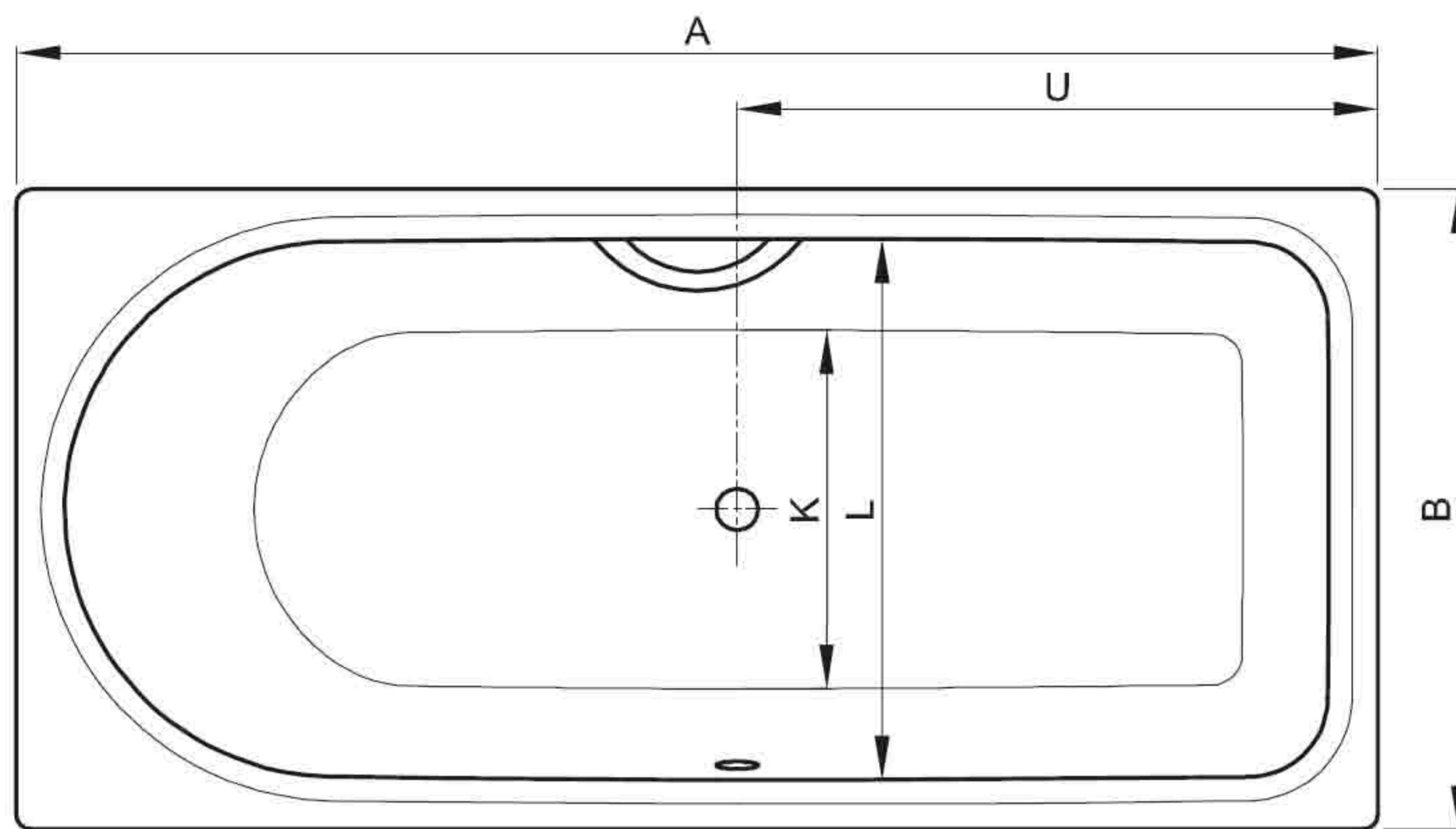
Výkres 170 x 80 cm, strana nohou vpravo, přepad vpředu, obj. č.: 8831, 8833, 8836, 8837, 8839
