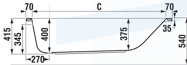
Instalační rozměry vany s panelem
