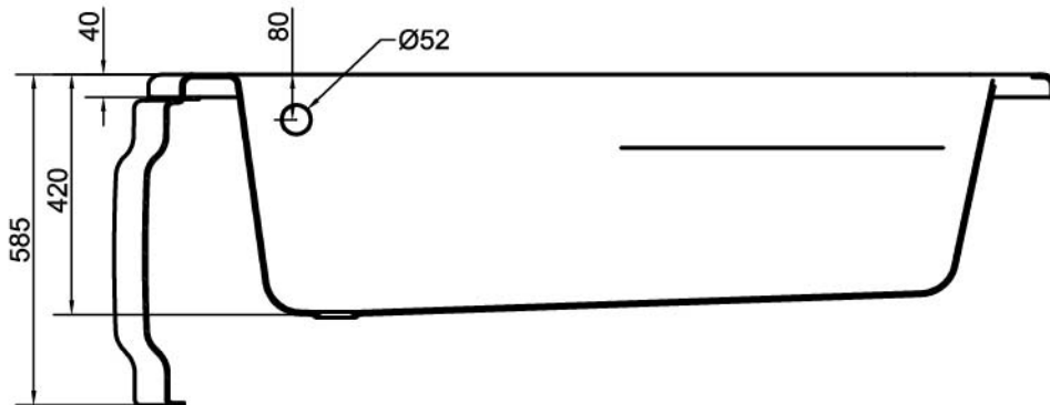
A-A (1 : 10)
