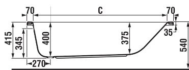
Instalační rozměry vany s panelem
