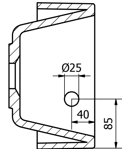
B-B ( 1 : 4 )
