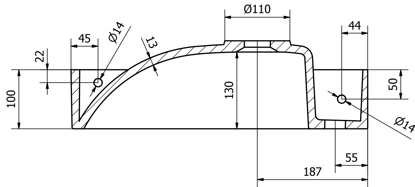
A-A ( 1 : 4 )
